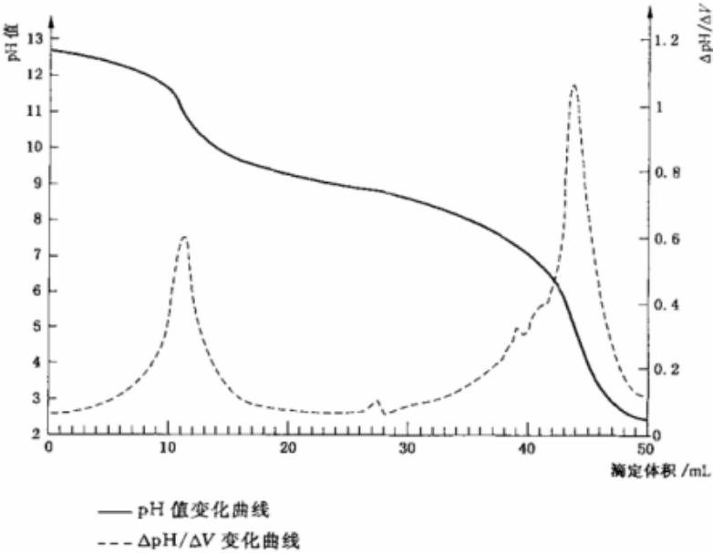
图 B.1 滴定及相关量的变化曲线
